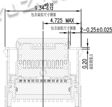
SECTION A-A(SC 1:1)
